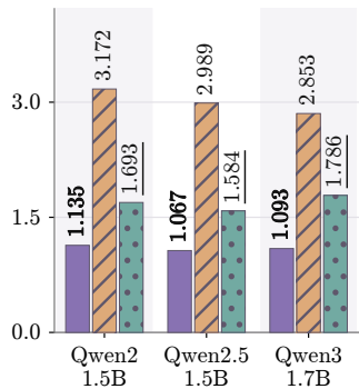
(a) KL ↓
