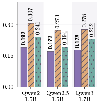
(b) Wasserstein ↓
