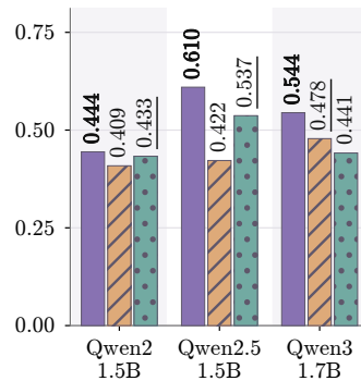
(d) Macro-F1 ↑
